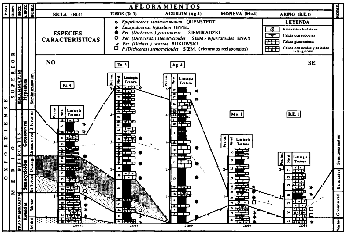
Figura 2.—Correlación bioestratigráfica de las columnas estudiadas. Mediante signos se indica la posición de las especies índice más importantes. La Subbiozona Stenocycloides se acuña hacia el Sureste (Plataforma de Arcos). La asociación de Perisphinctes (Dichotomoceras) stenocycloides SIEMIRADZKI-bifurcatoides ENAY, en Moneva y Ariño, está formada por elementos reelaborados (W). Figure 2.—Biostratigraphic correlation of the studied sections. The signs indicate the location of the most important species-index. The Stenocycloides Subbiozone decrease towards SE (Arcos Platform). The Perisphinctes (Dichotomoceras) stenocycloides SIEMIRADZKI-bifurcatoides ENAY assemblage is composed of reworked elements at Moneva and Ariño.
