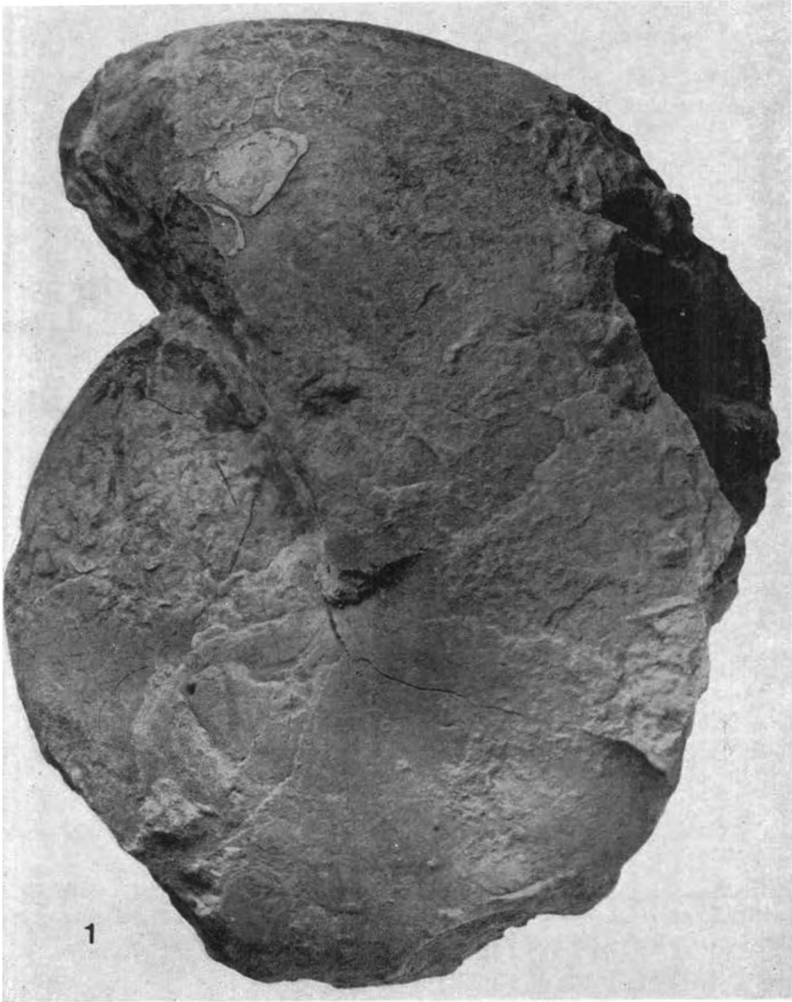
Fig. 1, Mayaites (Araucanites) reyesi West. et Ricc., subgen. et sp. nov., complete specimen, lateral view, \times 1 (MLP 12212). Plicatilis (? U. Cordatum) Zone, Aguada de la Mula, Sierra de Reyes
