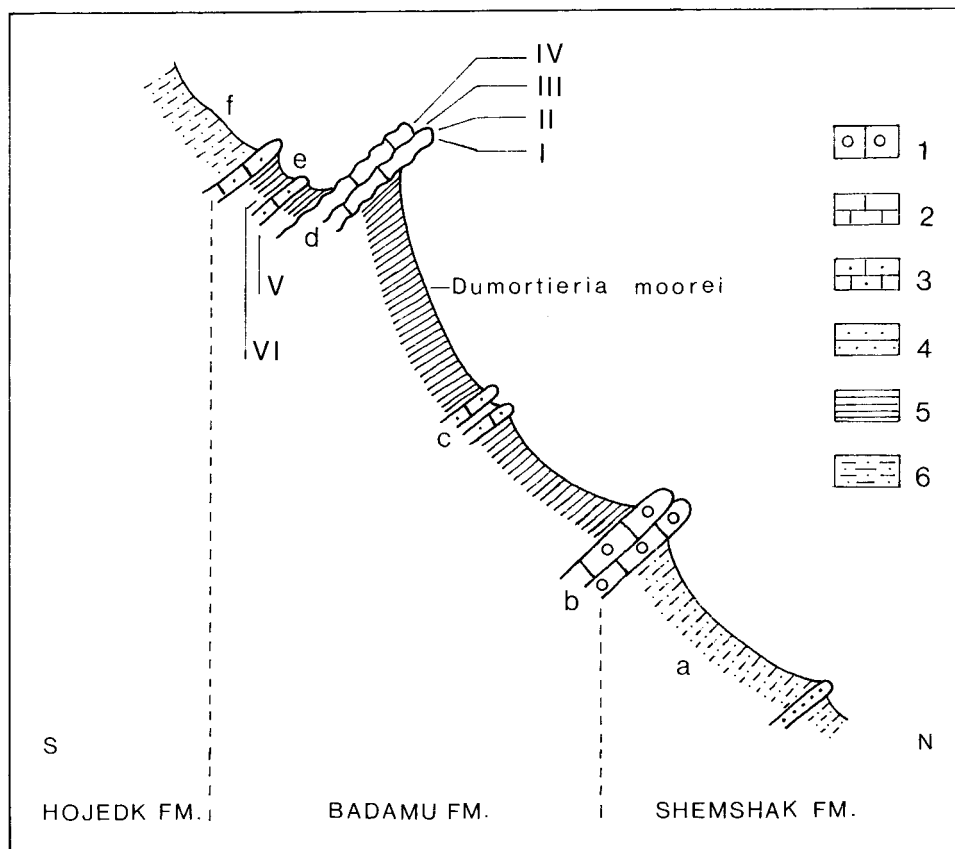
Abb. 2: Schematisiertes Profil durch die Badamu-Formation im Sarchtal, ca. 8 km WSW Ravar. a – f: s. Profilbeschreibung S. 14. 1: oolithischer Kalk; 2: knolliger Kalk; 3: sandiger Kalk; 4: Sandstein; 5: Mergel; 6: Schiefertone, Siltstein. I: Leioceras comptum ; II: Tmetoceras scissum ; III: Planammatoceras planiforme planum ; IV: Brasilia bradfordensis ; V: Kumatostephanus sp.; VI: Skirroceras sp. ex gr. S. macrum , Emileia sp. ex gr. E. polyschides .
