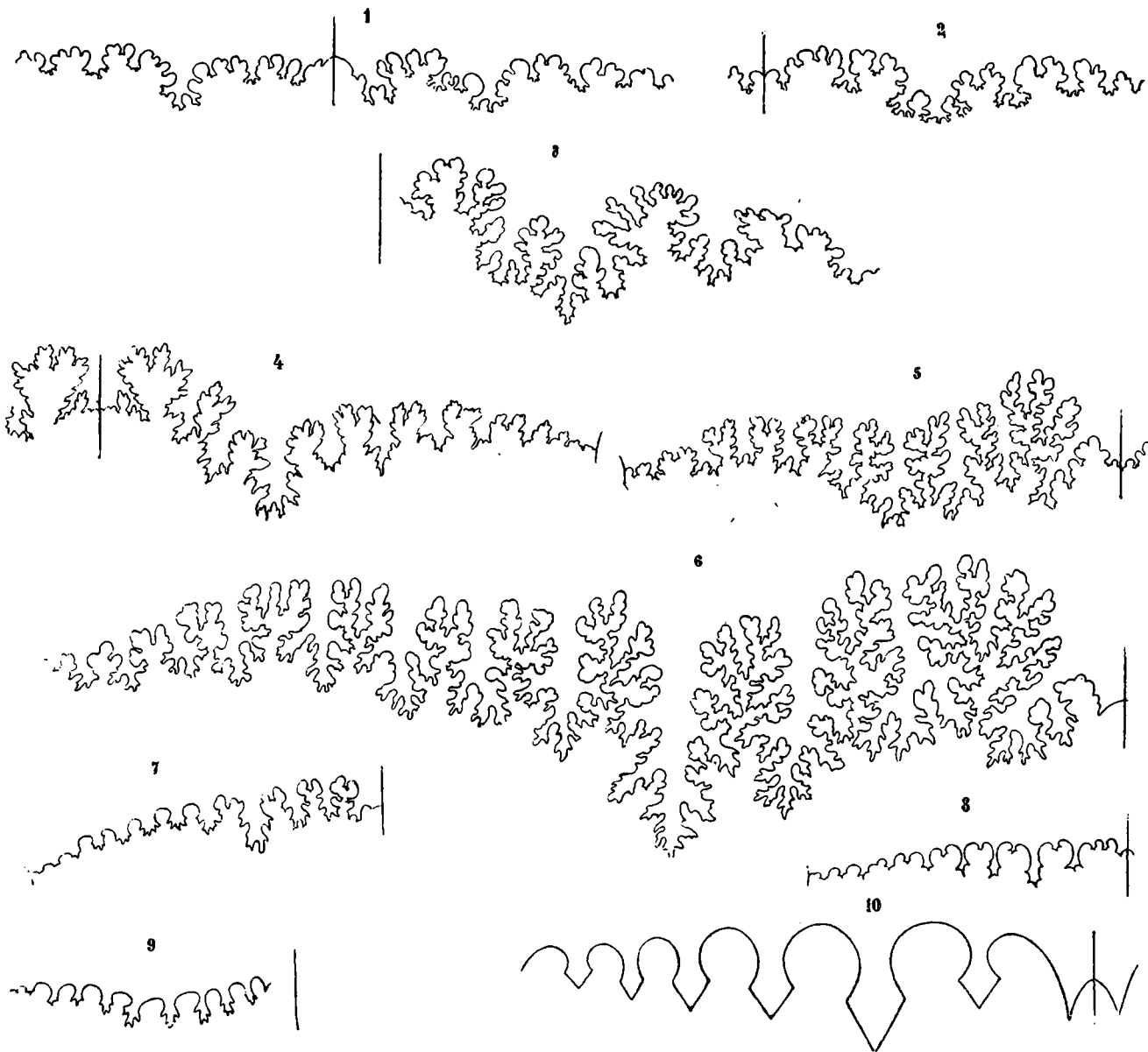
1. Oxynoticeras heteropleurum n. f. Hilsthon vom grossen Süntel. 2. Oxynoticeras Balduri Keyserling (Copie aus Petschoraland Tab. XIX, Fig. 6.) 3. Amaltheus clypeiformis Orb. aus dem Neocom von Escragnolles. 4. Sphenodiscus Guadeloupae (Römer?) Stoliczka (Copie aus Pal. Ind. Vol. I, Tab. XLVII, Fig. 20.) 5. Sphenodiscus syrtalis Mort. (Copie nach Schlüter, Cephalopoden der oberen norddeutschen Kreide, Tab. XV, Fig. 6.) 6. Sphenodiscus placenta Dek. (Copie nach Meek, Report on the United States geolog. survey of the territories. Vol. IX, pag. 466.) 7. Sphenodiscus lenticularis Owen. (Copie nach Meek, l. c. pag. 473.) 8. Engonoceras pierdenale Buch (Copie aus L. v. Buch, Ceratiten, Taf. VI, Fig. 10). 9. Engonoceras n. f. cf. Vibrayeum Orb. Cenoman von Tuffé, Dép. Sarthe. 10. Engonoceras Vibrayeumum . (Copie aus L. v. Buch, Ceratiten Tab. VII, Fig. 5.)
