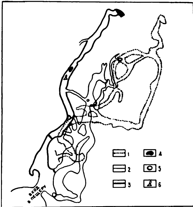
Схема ближней части Красных пещер (по В. Н. Дублянскому): 1 — 5-й этаж; 2 — 4-й и 3-й этажи; 3 — 2-й этаж; 4 — вода; 5 — крутой уступ (слева) и естественный колодец (справа); 6 — сталагмит «Гном».
