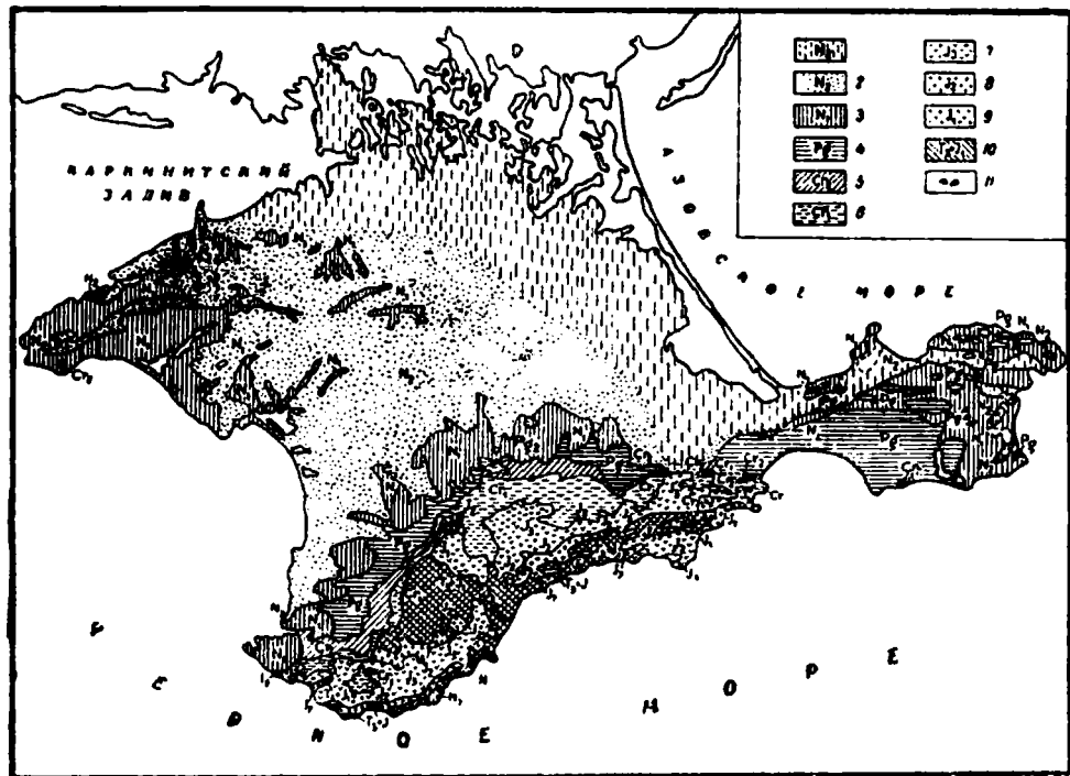
Схематическая геологическая карта Крыма. По М. В. Муратову.
