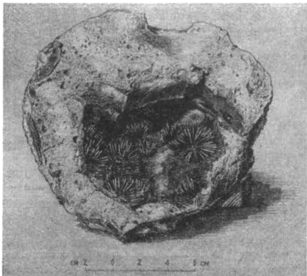
Конкреция из пласта керченской железной руды.
