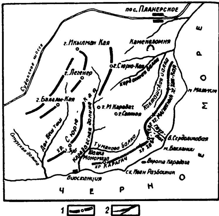
Схема хребтов, долин и бухт вулканической группы Кара-Дага. 1 — хребты; 2 — долины.
