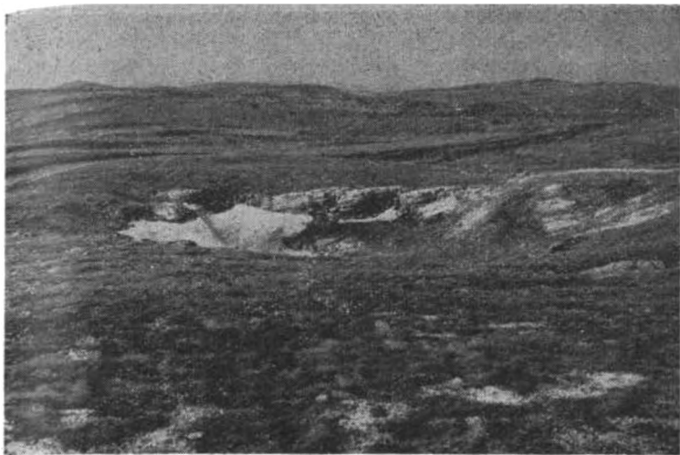
Карстовая впадина на Ай-Петринской яйле.
