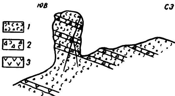
Геологический разрез скалы Сфинкс: 1 — зеленовато-бурый туф; 2 — туфобрекчия; 3 — поток сплитовой лавы.
