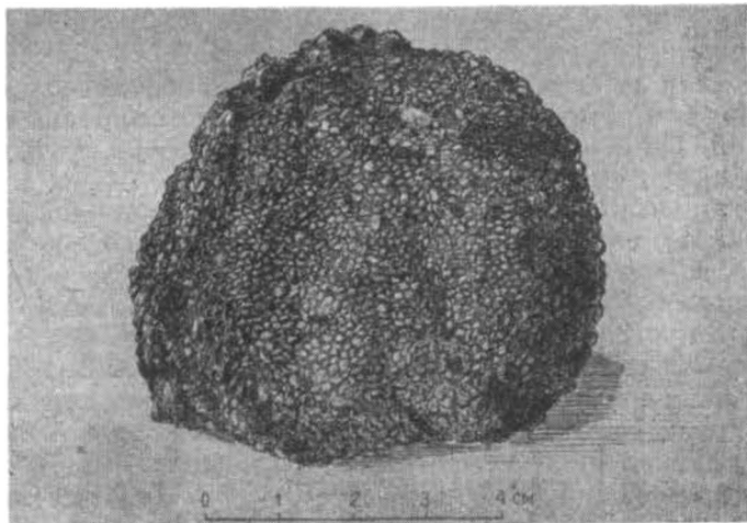
Керченская оолитовая руда.
