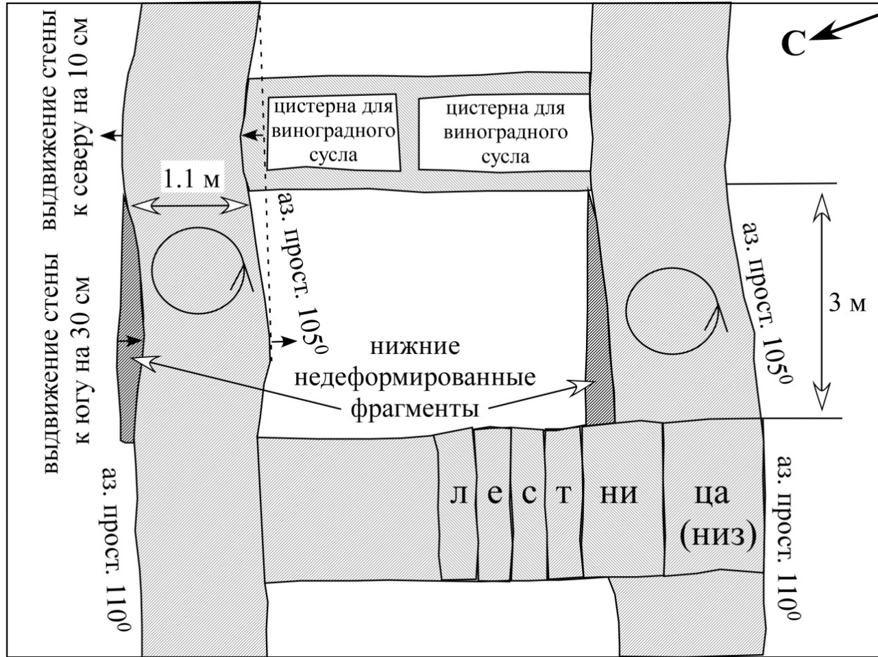
Рис. 9. Схематический план фрагмента северо-западного раскопа XXII (2 цистерны для виноградного сула). Видны развороты субмеридиональных стен против часовой стрелки в своей средней и верхней частях.
