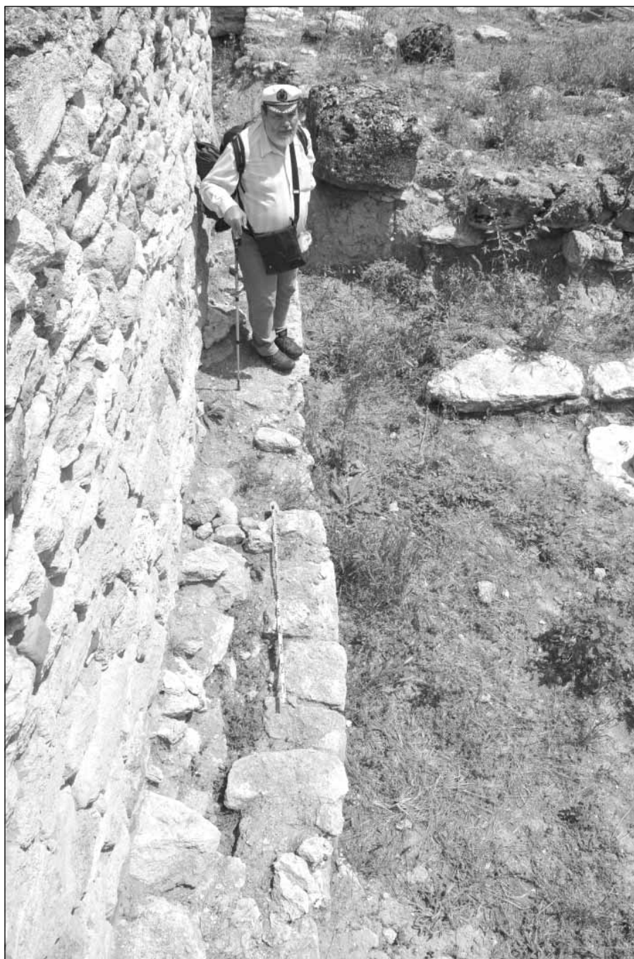
Рис. 6. Выдвижение к югу нижней части каменной кладки городской стены в раскопе XXVIII. Вид на восток.
