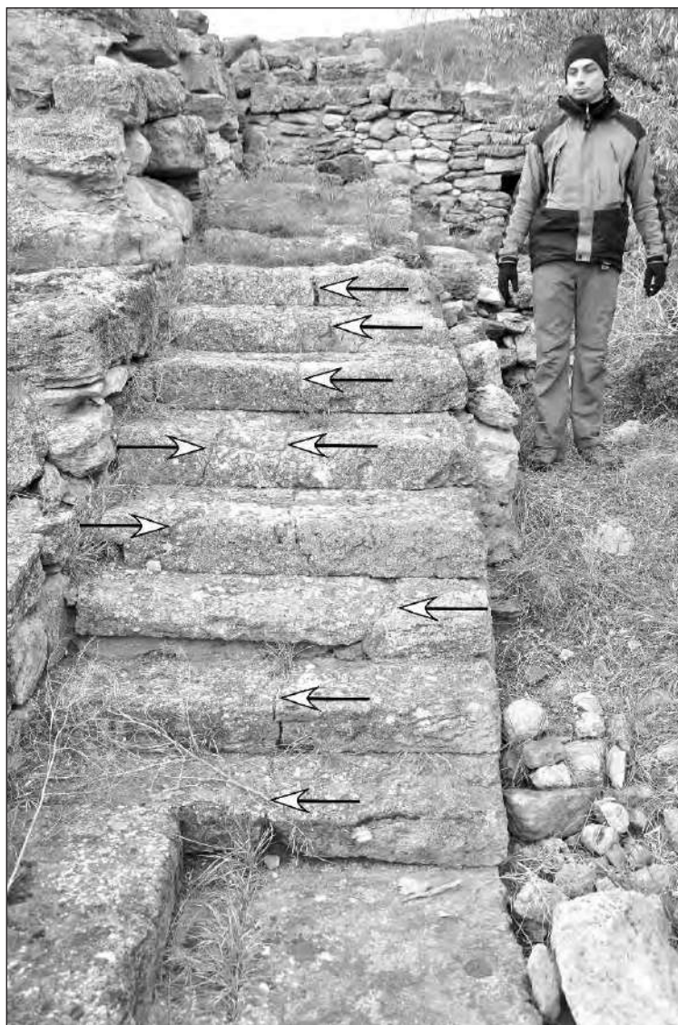
Рис. 13. Нимфей. Участок «М». Сквозные трещины через несколько строительных блоков в одной из лестниц IV в. до н.э.
