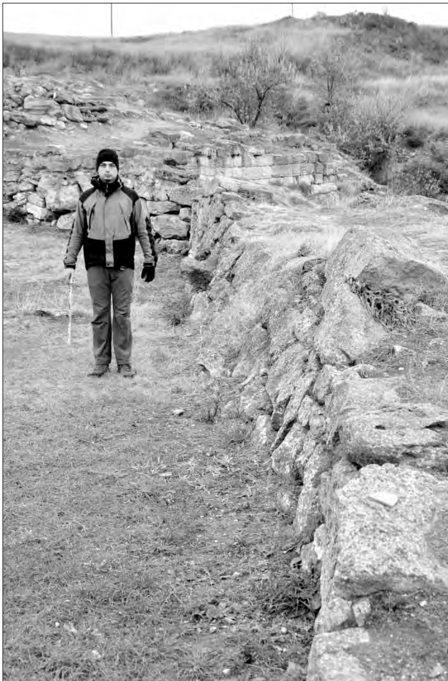
Рис. 4. Нимфей. Участок «М». Городская стена Нимфея с азимутом простирания 45–50° наклонилась на ЮВ под углом до 45° в верхней своей части, вид на СВ. Третья куртина оборонительной стены I – середины II вв. н.э.
