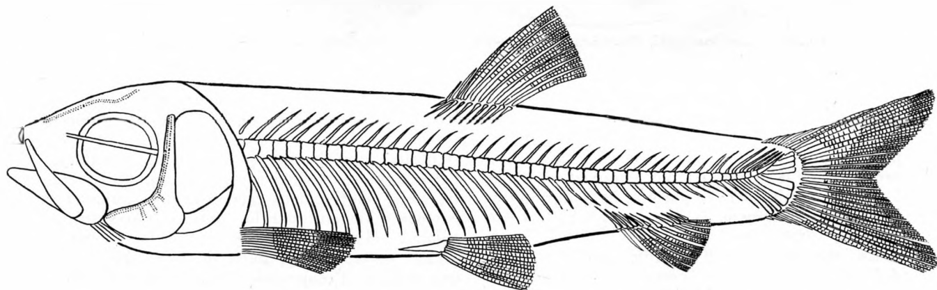
FIG. 3. — Manchurichthys uwatokoi SAITO. Reconstitution du corps (principalement d'après TAKAI [1943, fig. 12]).
