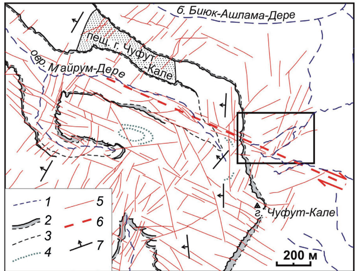
Ориентировка и тип основных групп трещин
