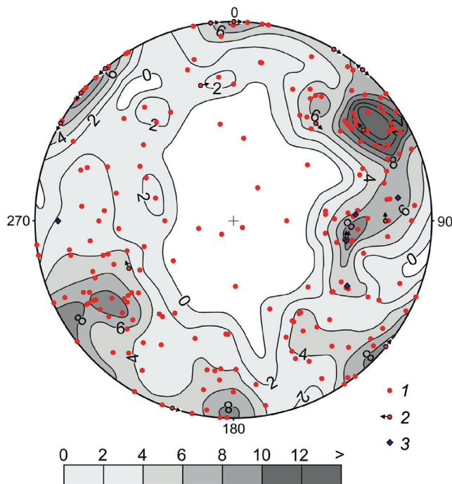
Рис. 4. Ориентировки трещин в стереографической проекции (верхняя полусфера): 1 — сколы с неустановленными смещениями, 2 — сколы с установленными смещениями, 3 — стилизованные поверхности трещин
