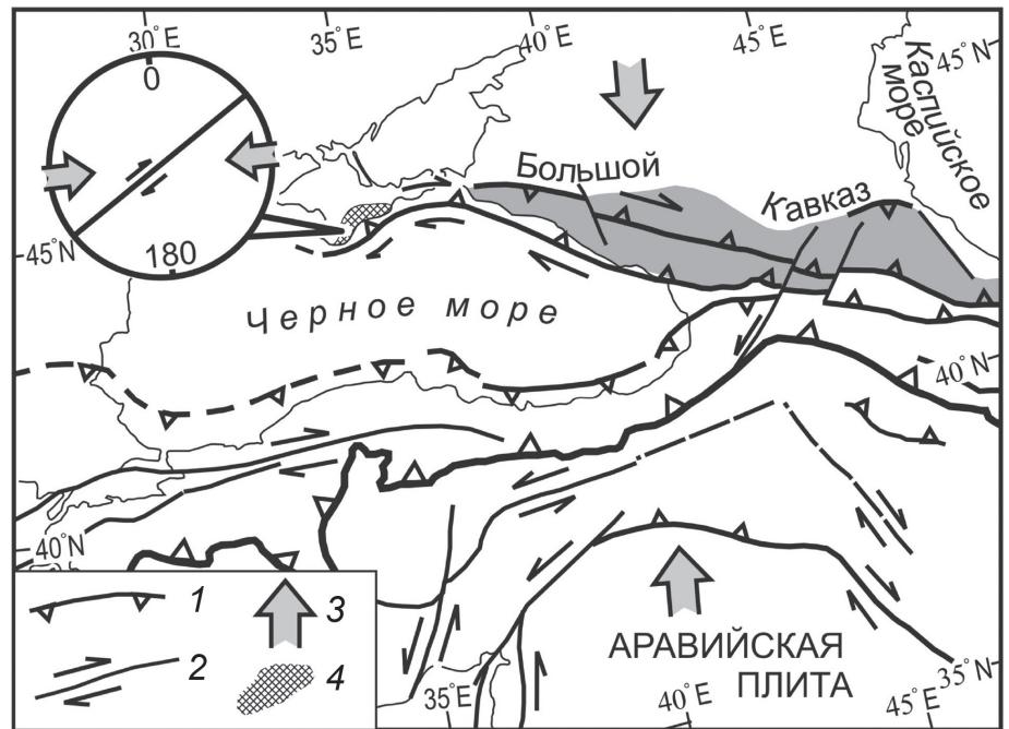
Рис. 6. Механизм возникновения в Горном Крыму транспрессии с эффективным субширотным сжатием (тектоническая схема по [Rolland et al., 2009] с изменениями): 1 — главные надвиги, 2 — сдвиги и сдвиговая составляющая разломов, 3 — напряжения сжатия, 4 — зона возникновения транспрессии в Горном Крыму
