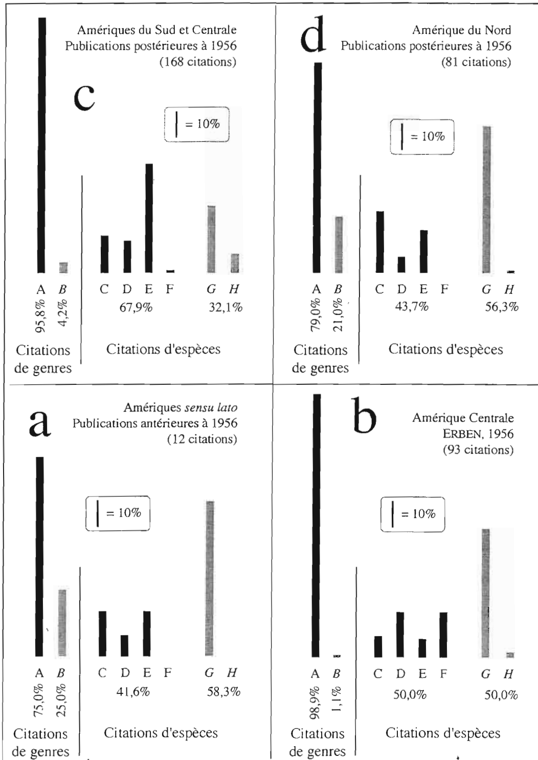
Fig. 5: Comparaison des principales pratiques taxinomiques appliquées aux faunes d'ammonites sinémuriennes d'Amérique du Nord d'une part et d'Amérique du Sud et Centrale d'autre part. Toutes les citations de la littérature accompagnées d'une illustration ont en principe été prises en compte. Les citations correspondant aux genres (A-B) et celles relatives aux espèces (C-H) sont décomptées et analysées indépendamment. A) pourcentage de citations de genres fondés sur des espèces-types téthysiennes ou nord-ouest européennes, B) pourcentage de citations de genres fondés sur des espèces-types américaines, C) pourcentage de citations d'espèces téthysiennes ou nord-ouest européennes, D) pourcentage de citations de formes rapprochées ( aff. ) d'espèces téthysiennes ou nord-ouest européennes, E) pourcentage de citations de formes rapprochées ( cf. ) d'espèces téthysiennes ou nord-ouest européennes, F) pourcentage de citations de formes considérées comme de simples sous-espèces locales d'espèces téthysiennes ou nord-ouest européennes, G) pourcentage de citations d'espèces américaines, H) pourcentage de citations de formes américaines considérées comme des espèces originales mais laissées en nomenclature ouverte.
