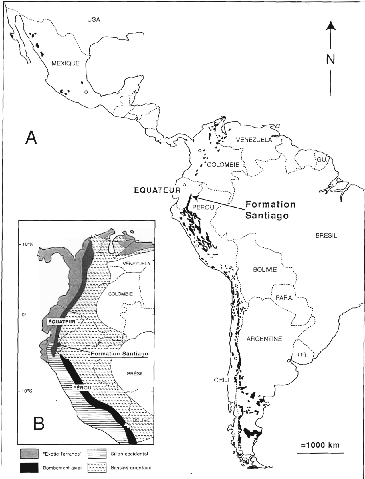
Fig. 1: Localisation de la Formation Santiago dans les cadres géographique et géologique d'Amérique du Sud et Centrale. A) Répartition des principaux affleurements du Jurassique en Amérique du Sud et Centrale [d'après WESTERMANN & RICCARDI (1990) et SMITH et al. (1994), modifié et complété]. B) Principales entités paléogéographiques pour le Mésozoïque de la partie septentrionale des Andes [d'après JAILLARD et al. (1995), modifié et complété].
