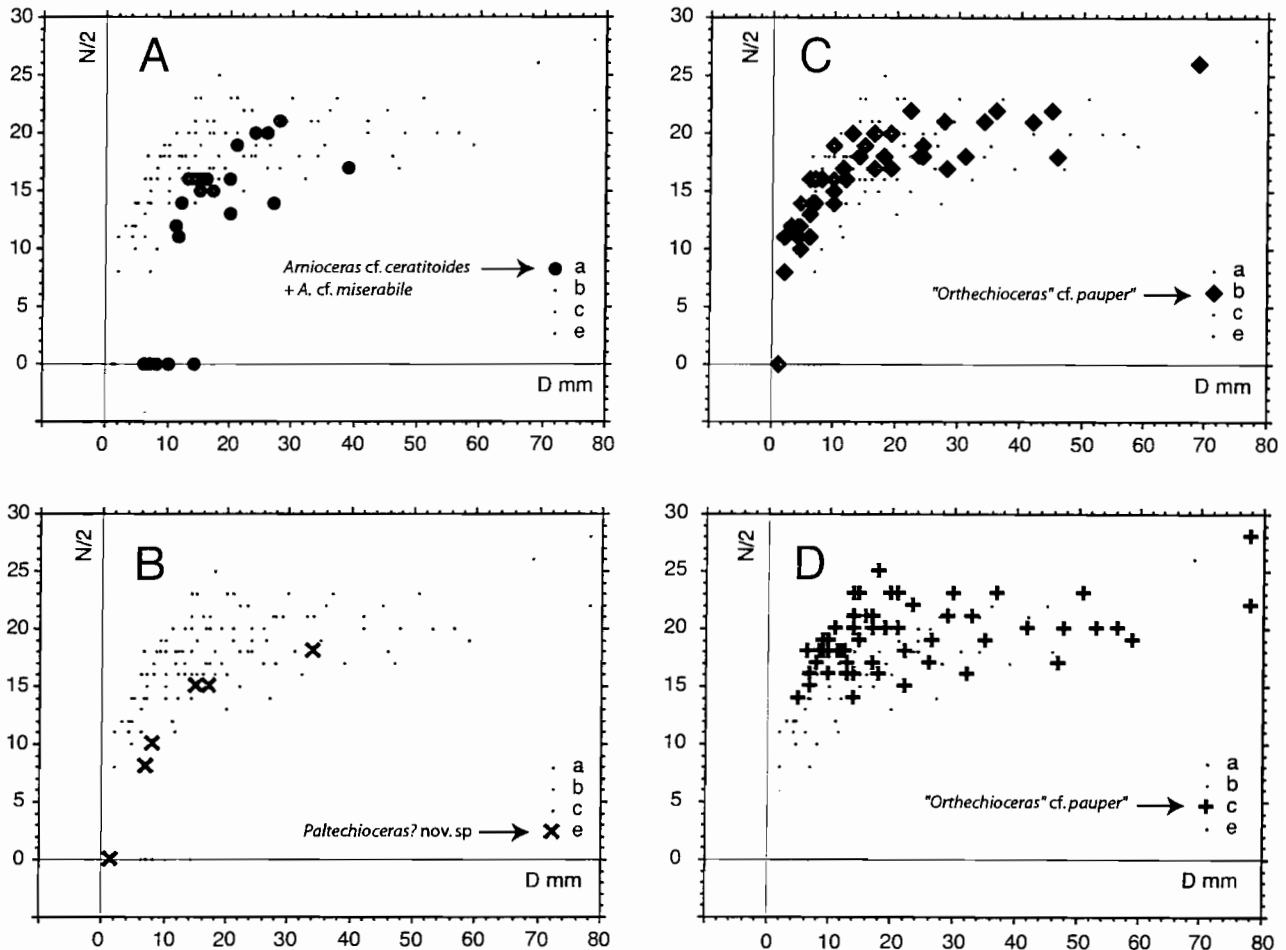
Fig. 3: Diagrammes de dispersion permettant de comparer la densité de costulation par demi-tour (N/2) en fonction du diamètre pour les espèces d'Arietitidae ( Arnioceras ) trouvés au point de récolte a et d'Echioceratidae (« Orthechioceras » récoltés en b et c, Paltechioceras? récoltés en e. Les petits points gris matérialisent le «pattern» de dispersion pour l'ensemble des espèces.
