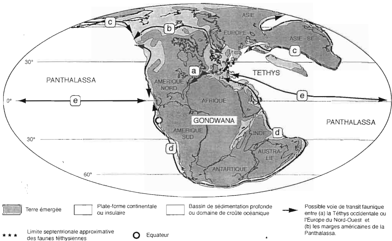
Fig. 4: Reconstitution paléogéographique globale d'après VRIELYNCK & BOUYSSÉ (2001, modifié) avec indication des principales voies possibles de transits fauniques entre la Téthys occidentale et ses confins nord-ouest européens d'une part et les marges américaines de la Panthalassa d'autre part. a) «Corridor hispanique», b «Corridor viking» et mers arctiques, c) voie péri-asiatique, d) voie péri-gonwanienne, e) voie «pantropicale».
