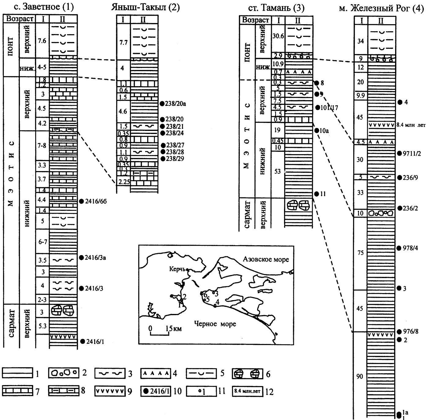
Рис. 1. Схема расположения изученных разрезов верхнемиоценовых отложений Керченского и Таманского полуостровов:
