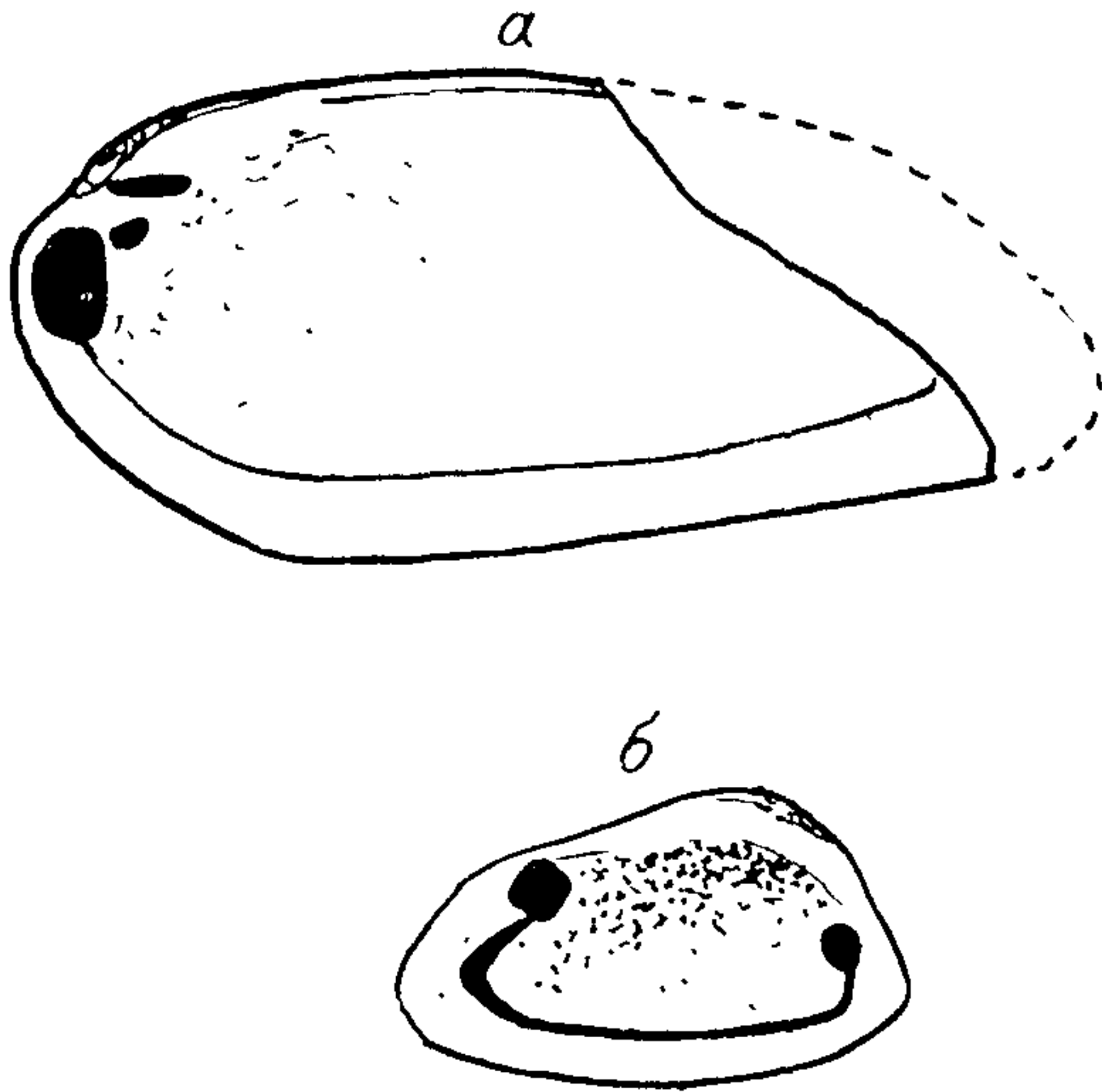
Рис. 12. Схематический рисунок правой (а) и левой (б) створок Permorphorus vendiavkiriensis sp. nov.
