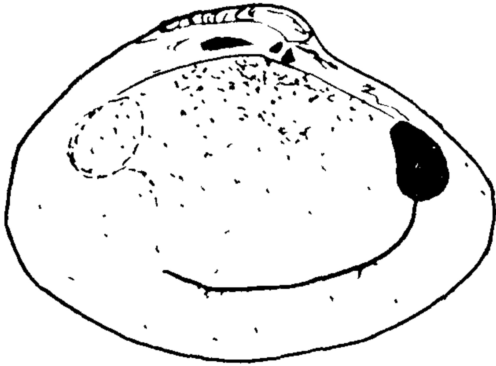
Рис. 16. Схематический рисунок правой створки Tancredia tuchkovi Kipar
