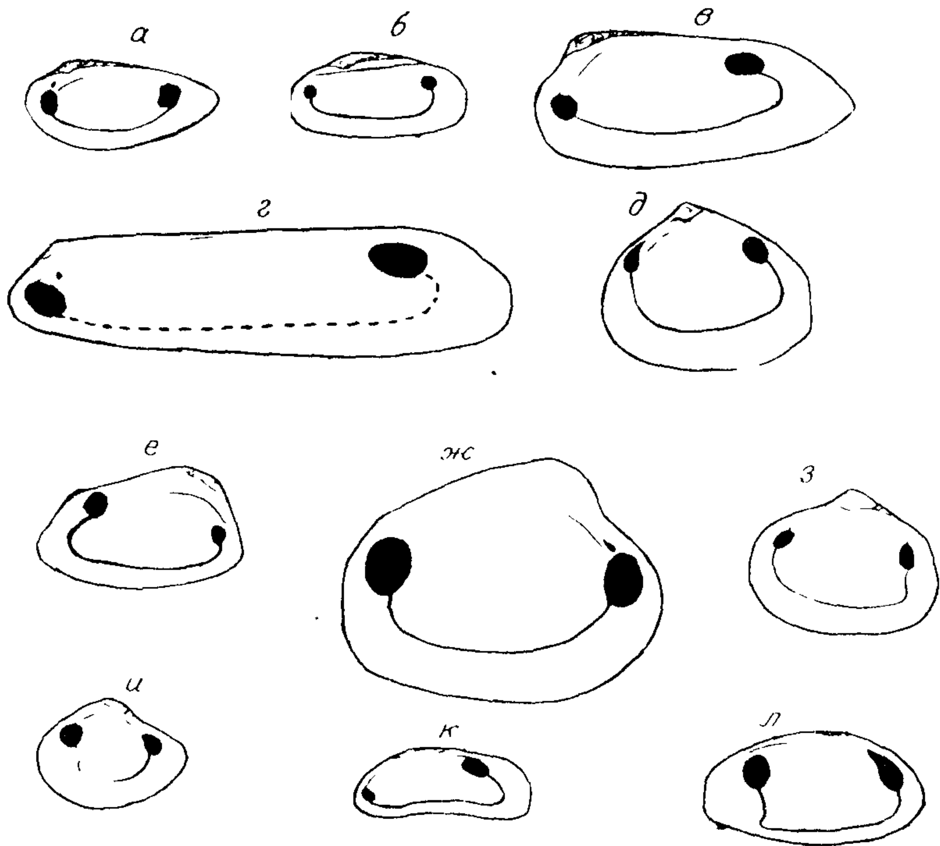
Рис. 3. Мускульные отпечатки и мантийная линия Cardinioides (а), Unionites (б), Janajia (в), Palaeopharus (г), Neoschizodus (д), Permophorus (е), Cardinia (ж), Pseudocorbula (з), Tancredia (и), Hiatella (к) и Panopea (л). Ум. 3/4.
