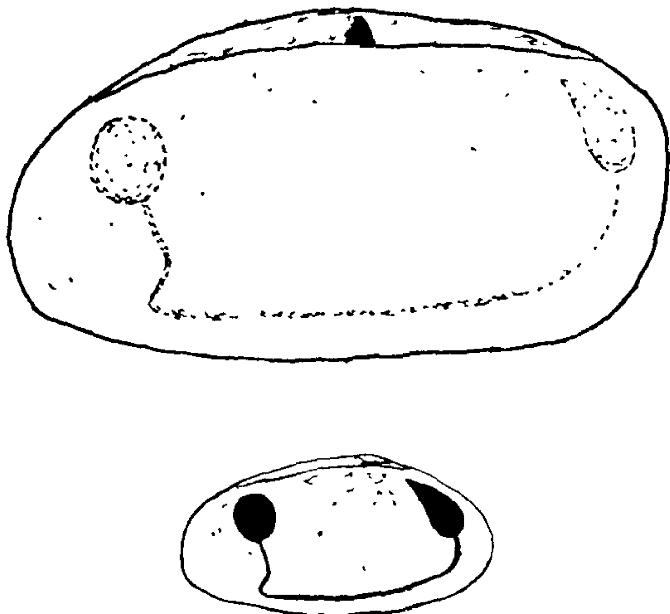
Рис. 18. Схематический рисунок левых створок Rapora anabarica sp. nov.
