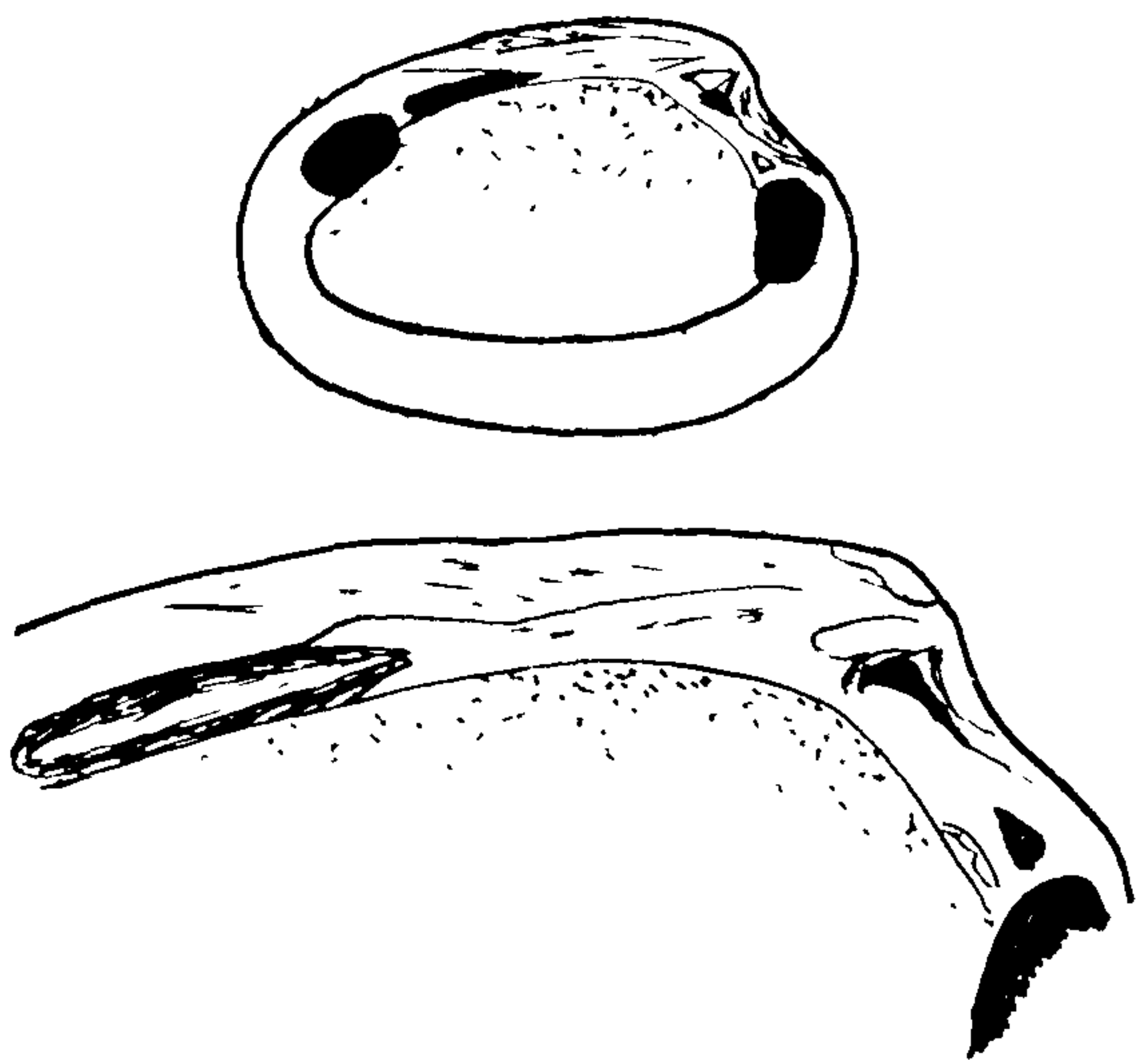
Рис. 13. Схематический рисунок левых створок Cardinia borealis Kipar.
