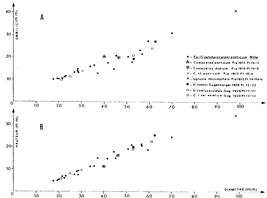
Fig. 2. Diagrammes de dispersion: A = croissance de l'ombilic en fonction du diamètre; B = croissance de la hauteur en fonction du diamètre.
